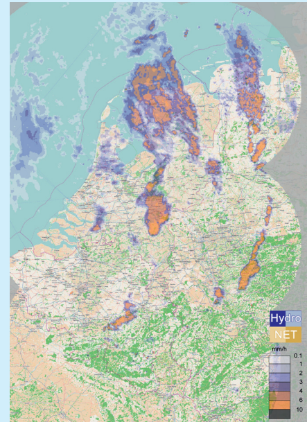
Afb. 3: Het internationale composietbeeld van de vlakdekkende neerslag op 22 juni 2011 om 16:00 uur (in verband met bliksemnslag was radar Zaventem toen buiten gebruik).
